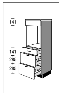
1475 mm SUBB S2A 148 600
