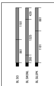
2051 mm BL SI3 75-200 BL SIK5NL 75-200 BL SIL5PK 75-200
