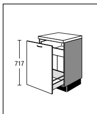
723 mm UAIS30 300 UAIS45 450 UAIS50 500 UAIS60 600
