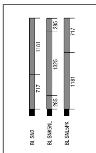
1907 mm BL SN3 75-200 BL SNK5NL 75-200 BL SNL5PK 75-200
