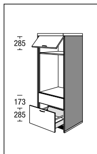
1475 mm SUGKA 65 148 650
