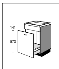
723 mm SPBA45 450 SPBA50 500 SPBA60 600
